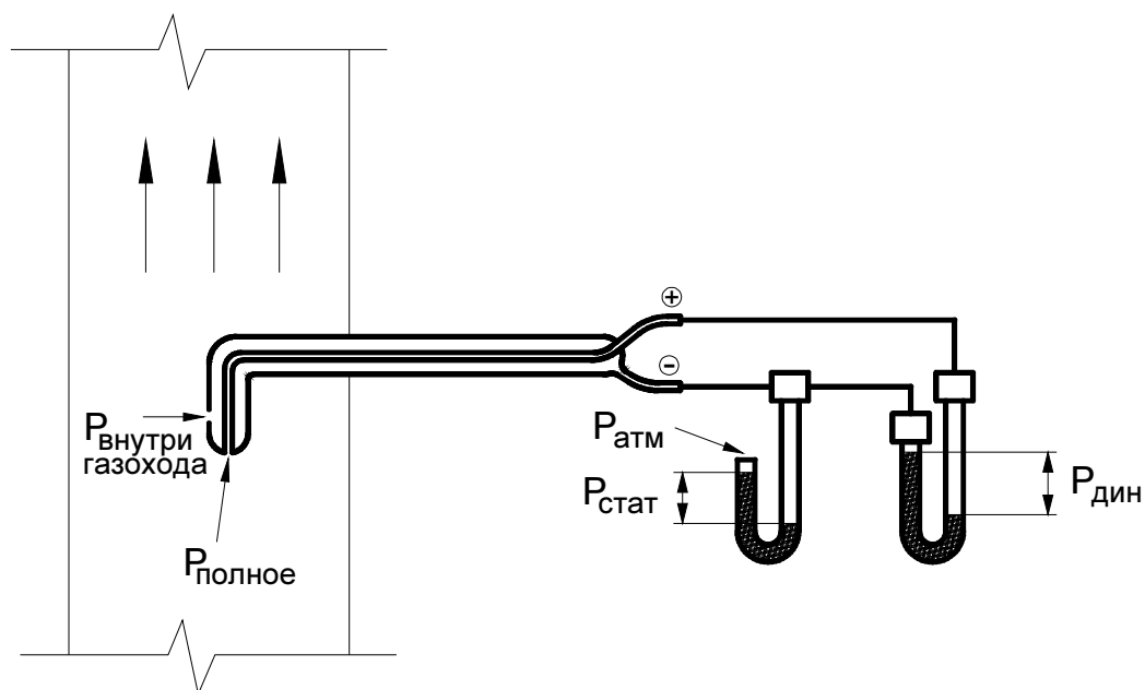
Рисунок 11. Размещение газонапорной трубки в газоходе
