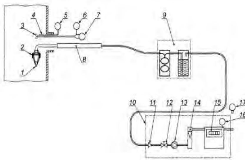
Рисунок 17. Пример системы отбора проб внутренней фильтрацией (фильтр внутри газохода)
